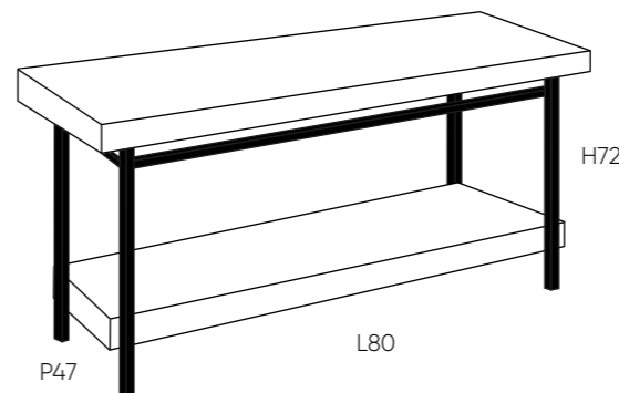
Metalna konstrukcija za nadgradni umivaonik s policom: HARMONY Metal structure for washbasin top with ledge: HARMONY
